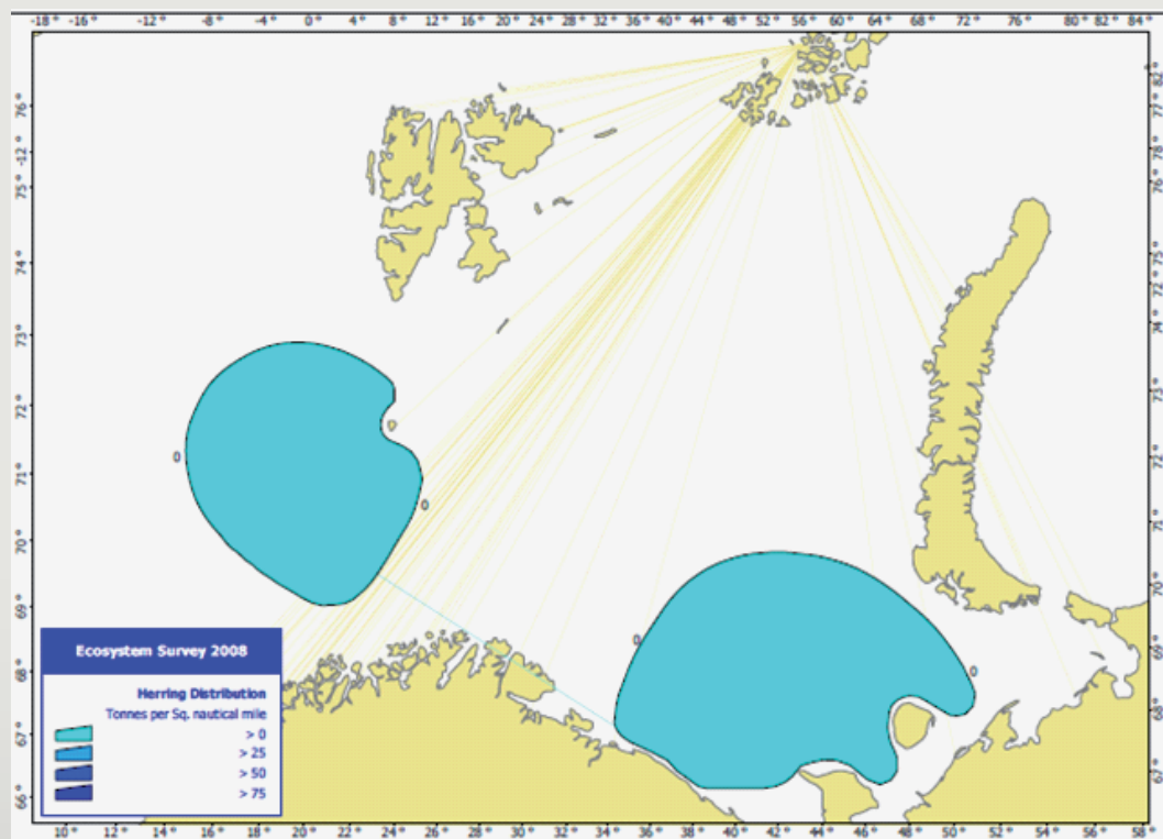
Figur 4.5.1.3 Estimert relativ akustisk tetthetsfordeling av sild i Barentshavet i 2008 (fra økosystemtøktet i august-oktober).
