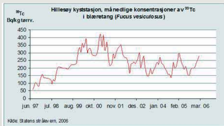
Figur 4.11.8.2 Tidsserie for ^{99}\text{Tc} i blæretang fra Hillesøy ( \text{Bq kg}^{-1} tørrvekt) i perioden 1997-2006.
