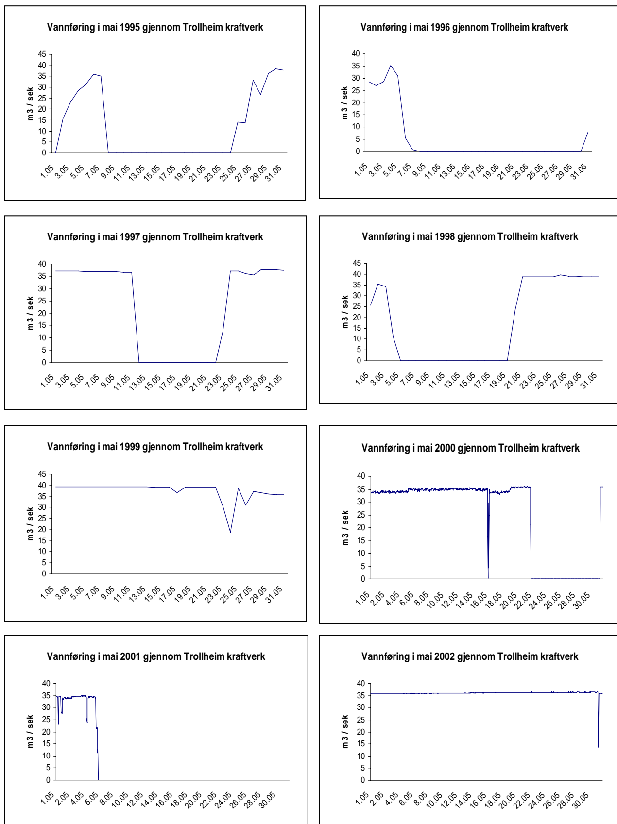
Figur 23. Driftsvannføring (på timebasis, m^3/s ) gjennom Trollheim kraftverk i mai i årene 1995-2004 (fortsettelse neste side).
