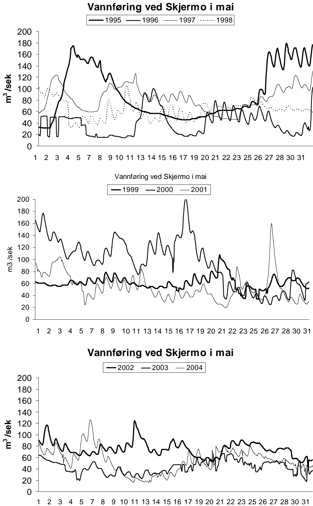
Figur 22. Vannføring (på timebasis, m³/s) målt ved Skjermo i mai i årene 1995-2004.
