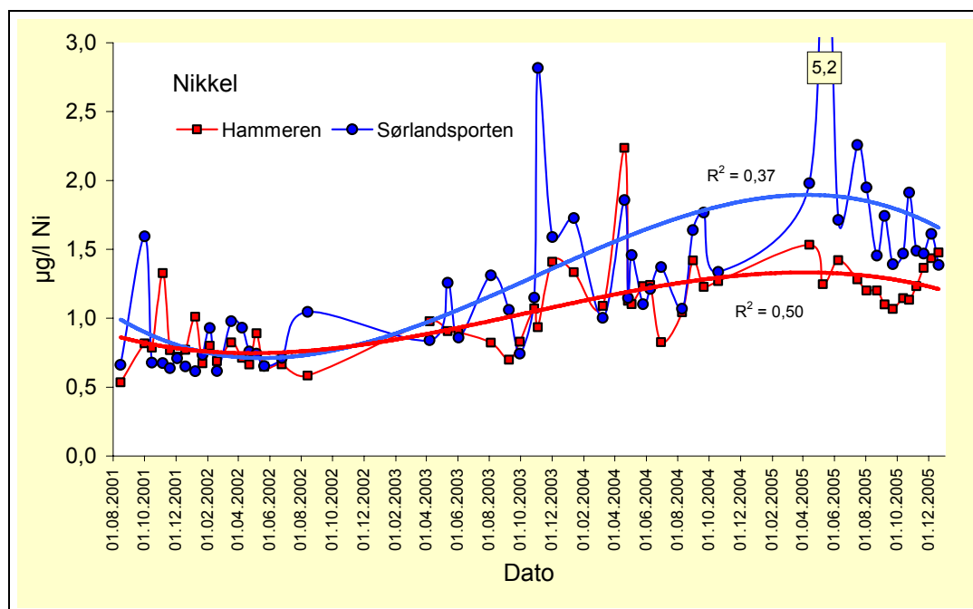
Figur 13. Nikkell (Ni) i Hammerbekken ved Hammeren, utløpet av Aklandstjern (E 18) og Molandsbekken ved Sørlandsporten i perioden august 2001 til desember 2005.
