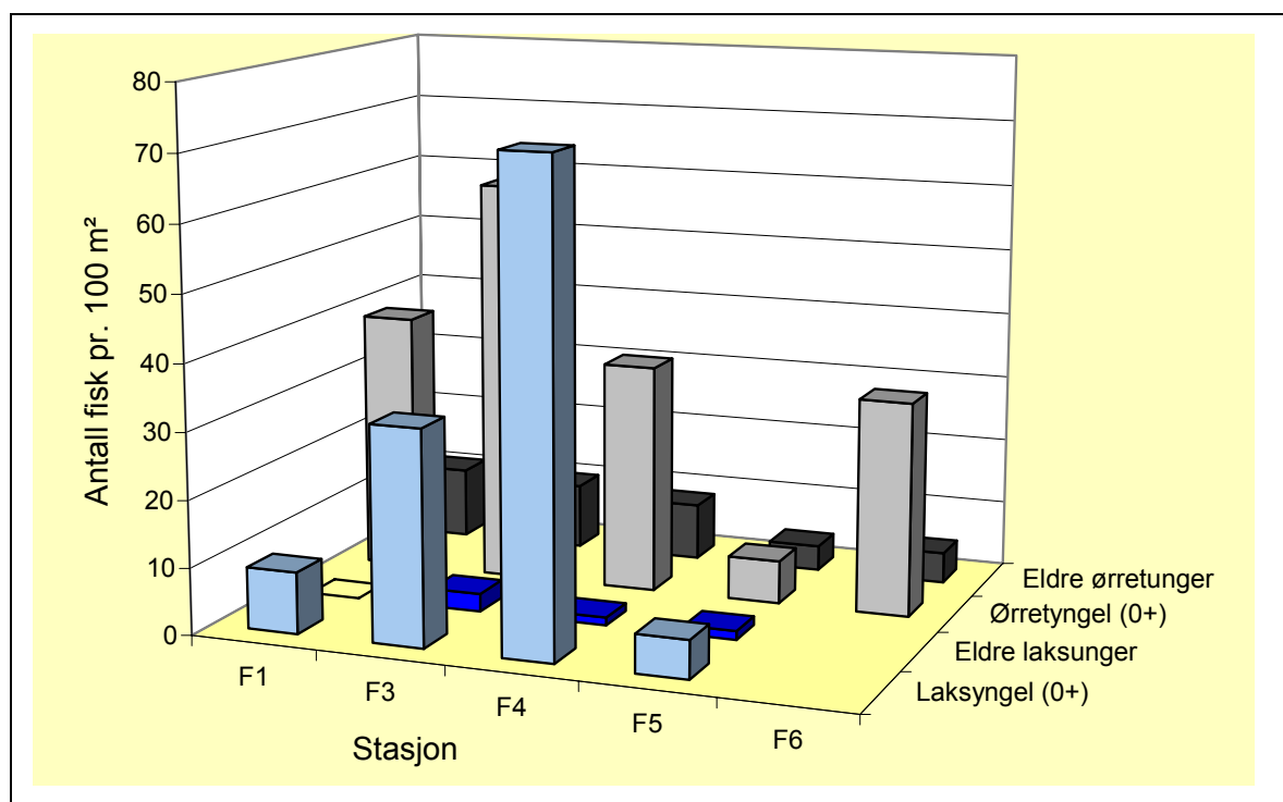
Figur 16. Tetthet per 100 m 2 av laks og ørret på fem stasjoner i Hammerbekken som ble undersøkt i august 2005. Stasjon F6 ligger ovenfor lakseførende strekning.
