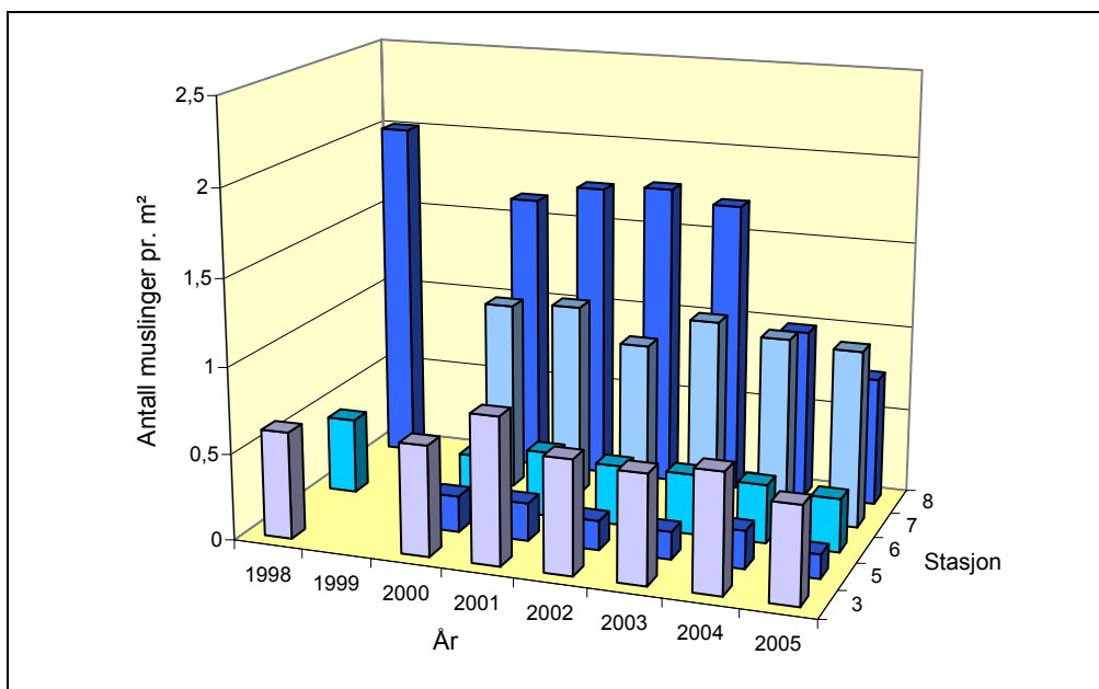
Figur 20. Antall levende elvemusling på utvalgte stasjoner i Hammerbekken som ble undersøkt i august 1998 og 2000-2005 basert på tellinger i transekter. Tetthet er oppgitt som antall muslinger per m 2 . Jf. Vedlegg 4. Stasjonenes beliggenhet er vist på figur 1.
