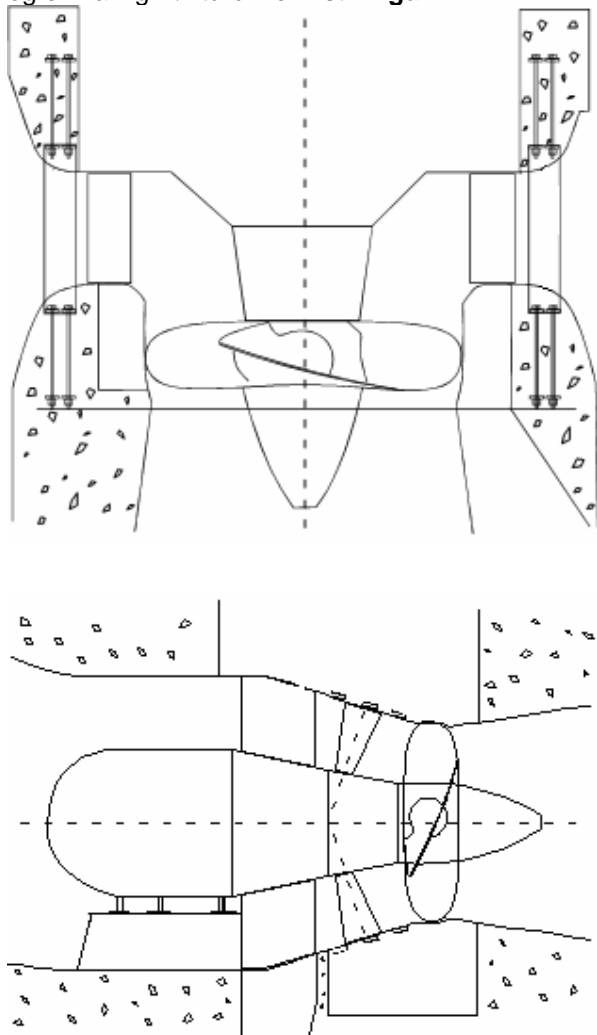
Figur 2. Prinsippskisse av Kaplan (øvre) og Rørturbin (nedre)
