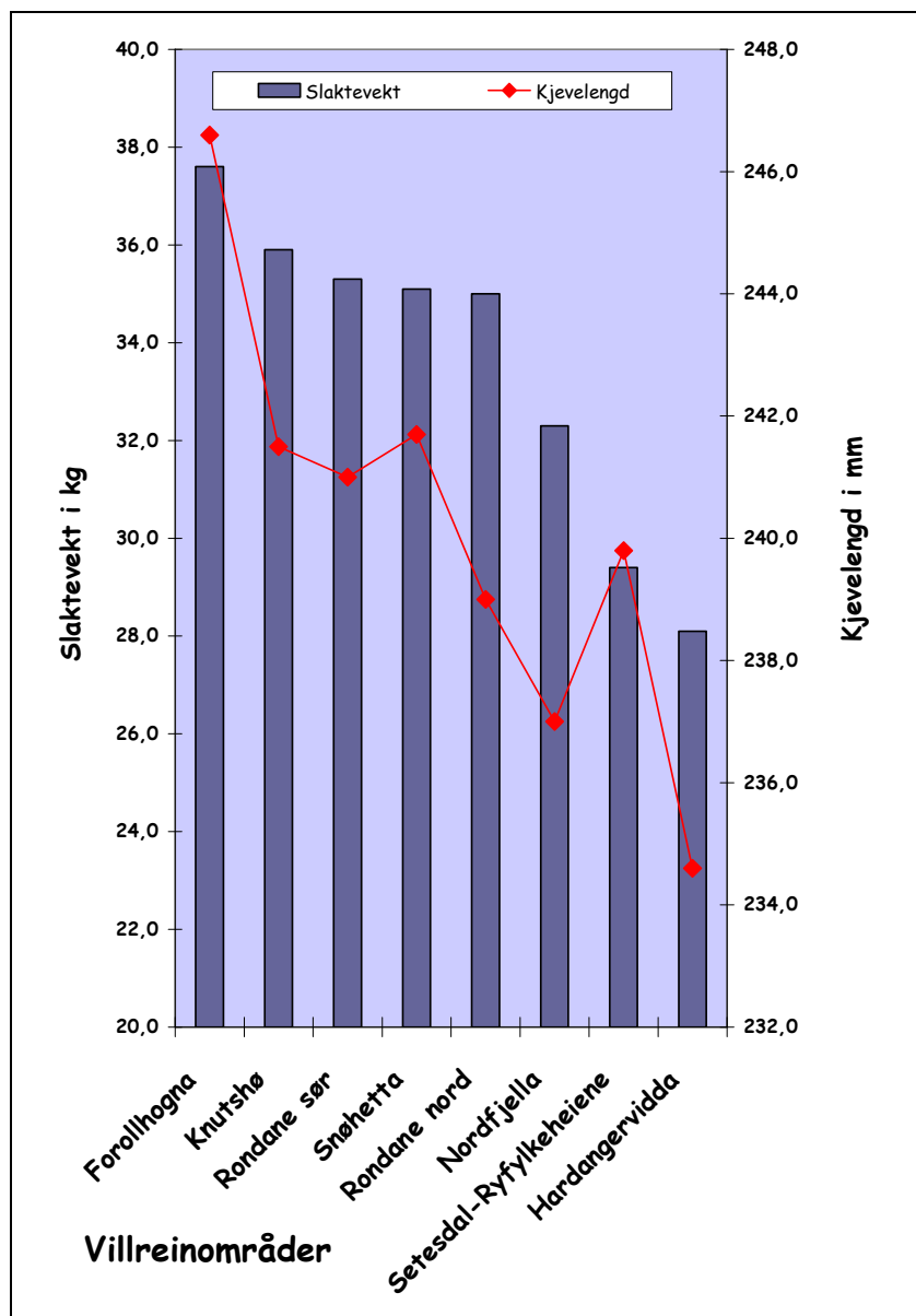
Figur 19. Kjevelengder og slaktevekt som mål på kondisjon i ulike norske villreinområde.
