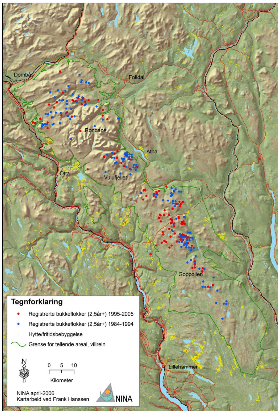
Figur 13. Lokalteter for observerte bukkeflokkar dei siste 22 åra (strukturteljingar på seinvintren). Hyttekonsentrasjonar framgår med gule felt. Kartgrunnlag: N250 fra Statens Kartverk. Bruksrett: Norge Digitalt, NINA
