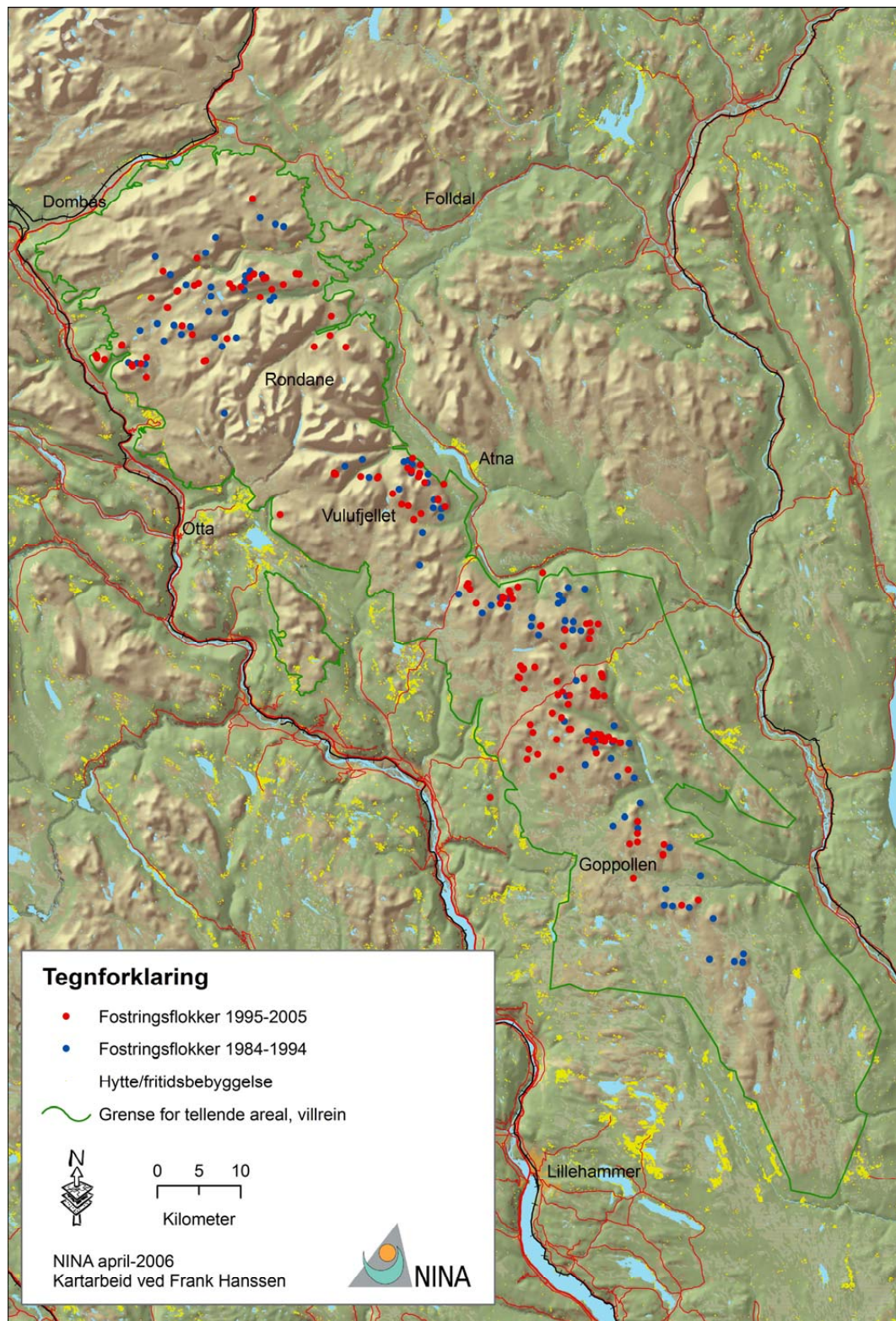
Figur 14. Lokaltetar for observerte fostringsflokkar dei siste 22 åra (struktureteljingar på sein-vinteren). Hyttekonsentrasjonar framgår med gule felt. Kartgrunnlag: N250 fra Statens Kartverk. Bruksrett: Norge Digitalt, NINA
