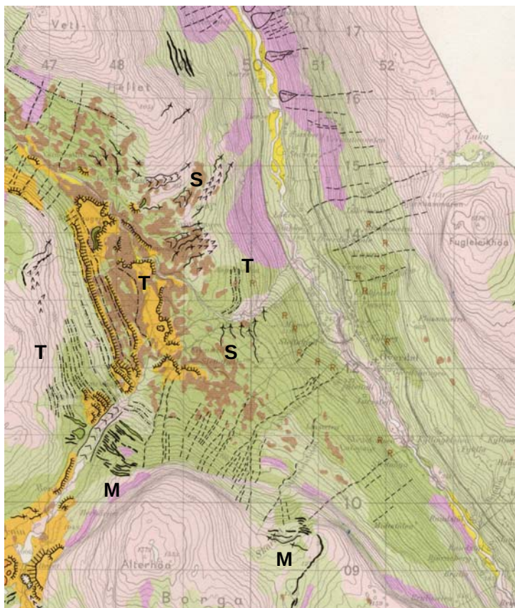
Figur 2. Kvartærgeologisk kart over undersøkelsesområdet med omgivelser (Sollid og Kristiansen 1984). Kartet viser stort kvartærgeologisk mangfold knyttet til bredemte sjøer, terrasser (T), spylereenner og spylefelt (S), og moreneformer (M). Quaternary map of the investigation area and surroundings (Sollid og Kristiansen 1984). The map show a large geodiversity especially linked to icedammed lakes (T), meltwater channels (S) and moraines (M).
