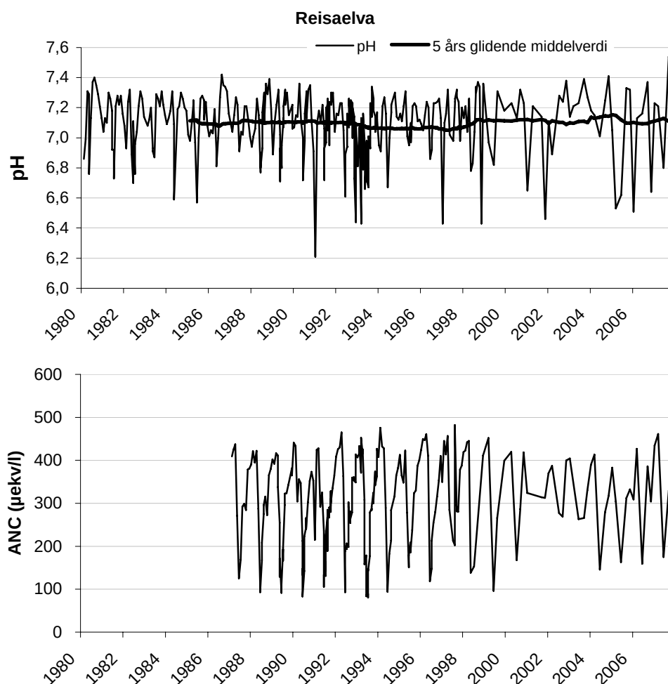
Figur 11. pH med 5 års glidende middelvei og ANC i Reisaelva i perioden 1980-2007.
