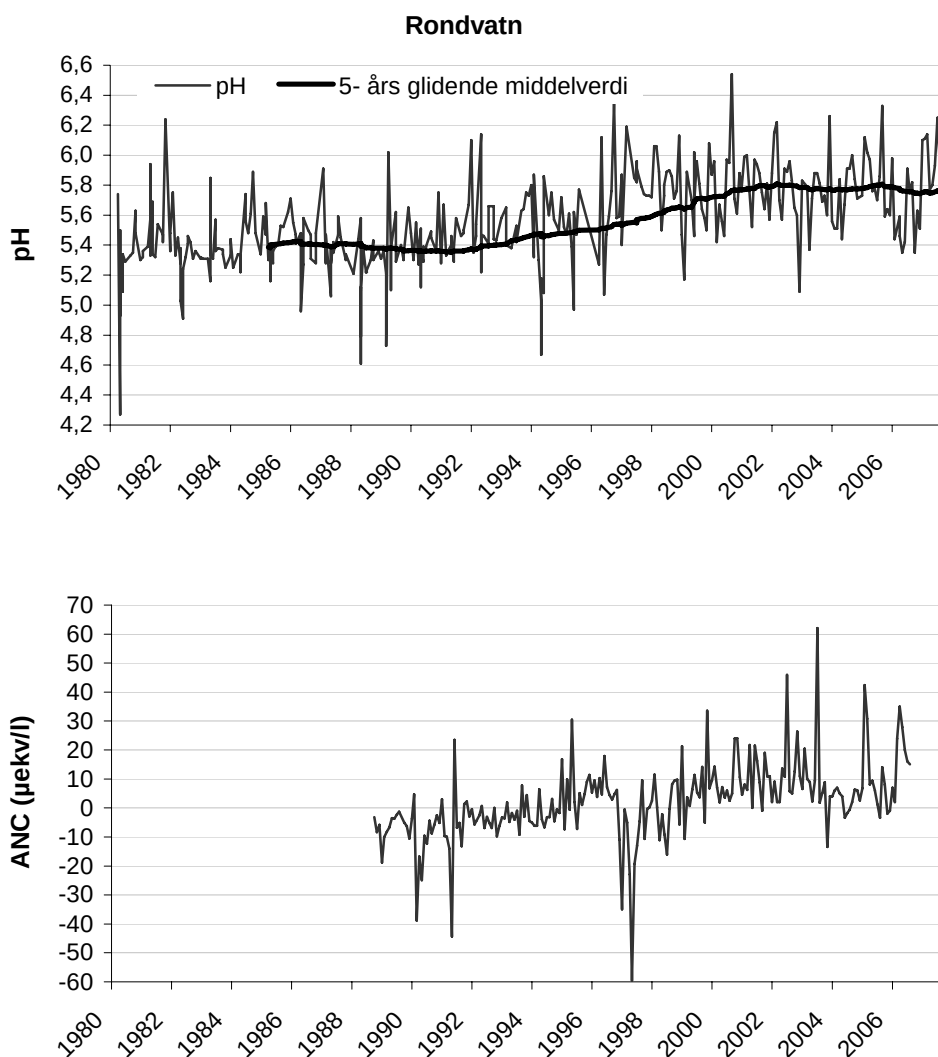
Figur 2. pH med 5 års glidende middelerdi og ANC i Rondvatn i perioden 1980-2007.
