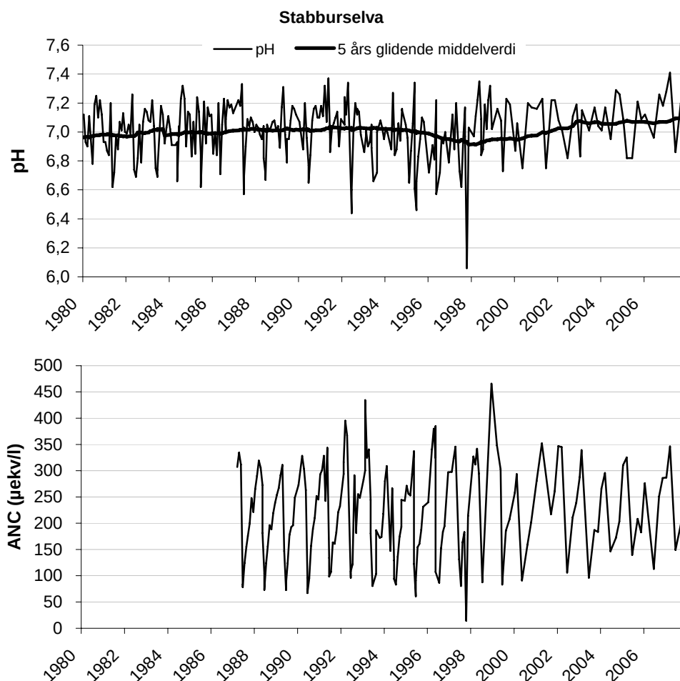
Figur 13. pH med 5 års glidende middelvei (dataserien starter i 1973) og ANC i Stabburselva i perioden 1980-2007.
