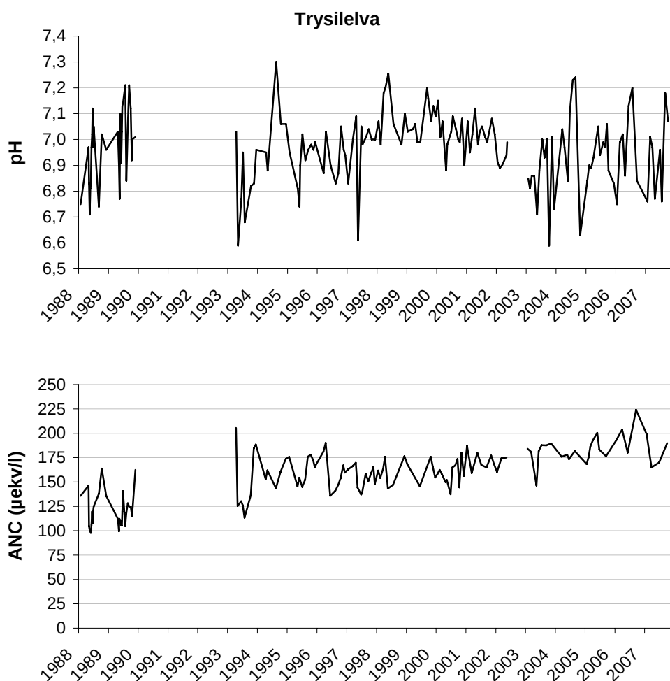
Figur 14. pH og ANC i Trysilelva i perioden 1988-2007.
