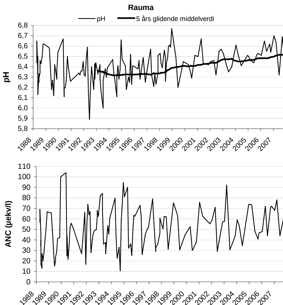
Figur 17. pH med 5 års glidende middelværdi og ANC i Rauma i perioden 1988-2007.
