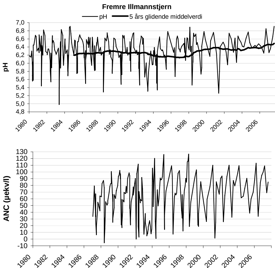
Figur 4. pH med 5 års glidende middelerdi og ANC i Fremre Illmannstjern i perioden 1980-2007.
