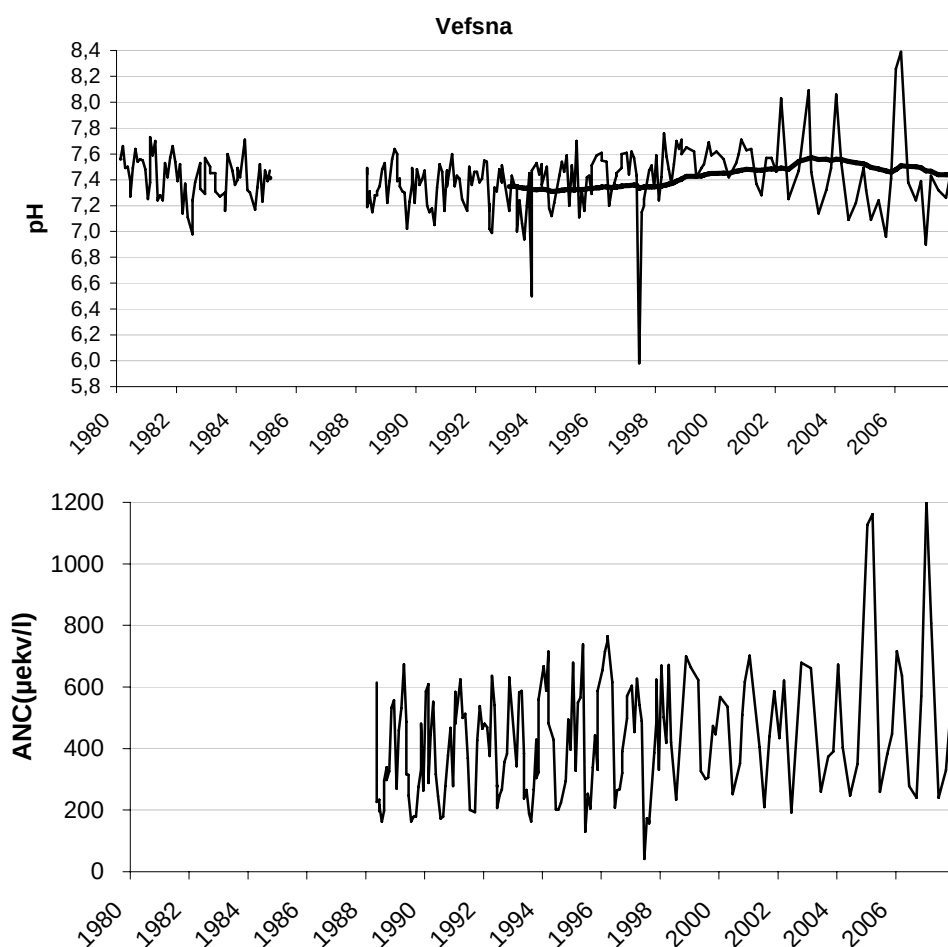
Figur 20. pH med 5 års glidende middelværdi (beregnet fra 1988) og ANC i Vefsna i perioden 1980-2007.
