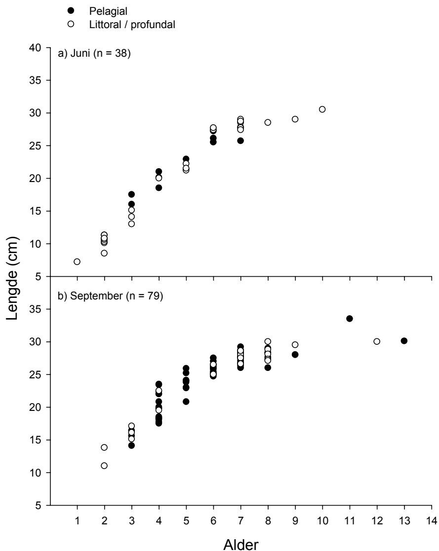
Figur 4.5 Forhold mellom alder og lengde til røye fanget på flytegard og bunngard ved prøvefiske i Storsjøen i a) juni og b) september.
