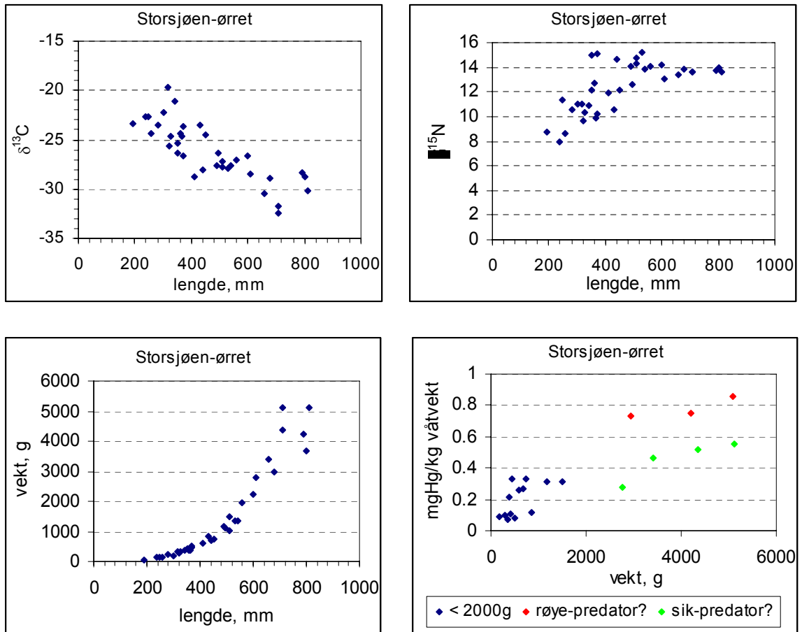
Figur 4.21 Sammenhengen mellom ørretens lengde og \delta^{13}C og \delta^{15}N (øvre paneler), mellom lengde og vekt, samt sammenhengen mellom vekt og kvikksølvkonsentrasjon (data fra 2001, Rognerud og Fjeld 2002)
