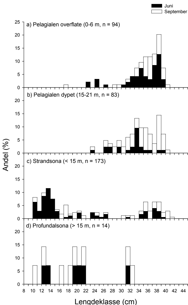
Figur 4.6 Lengdefordeling til sik fanget på flytegarn på a) 0-6 m dyp og b) 15-21 m dyp og med bunngarn i c) strandsona på bunngarn i profundalen (> 15 m).
