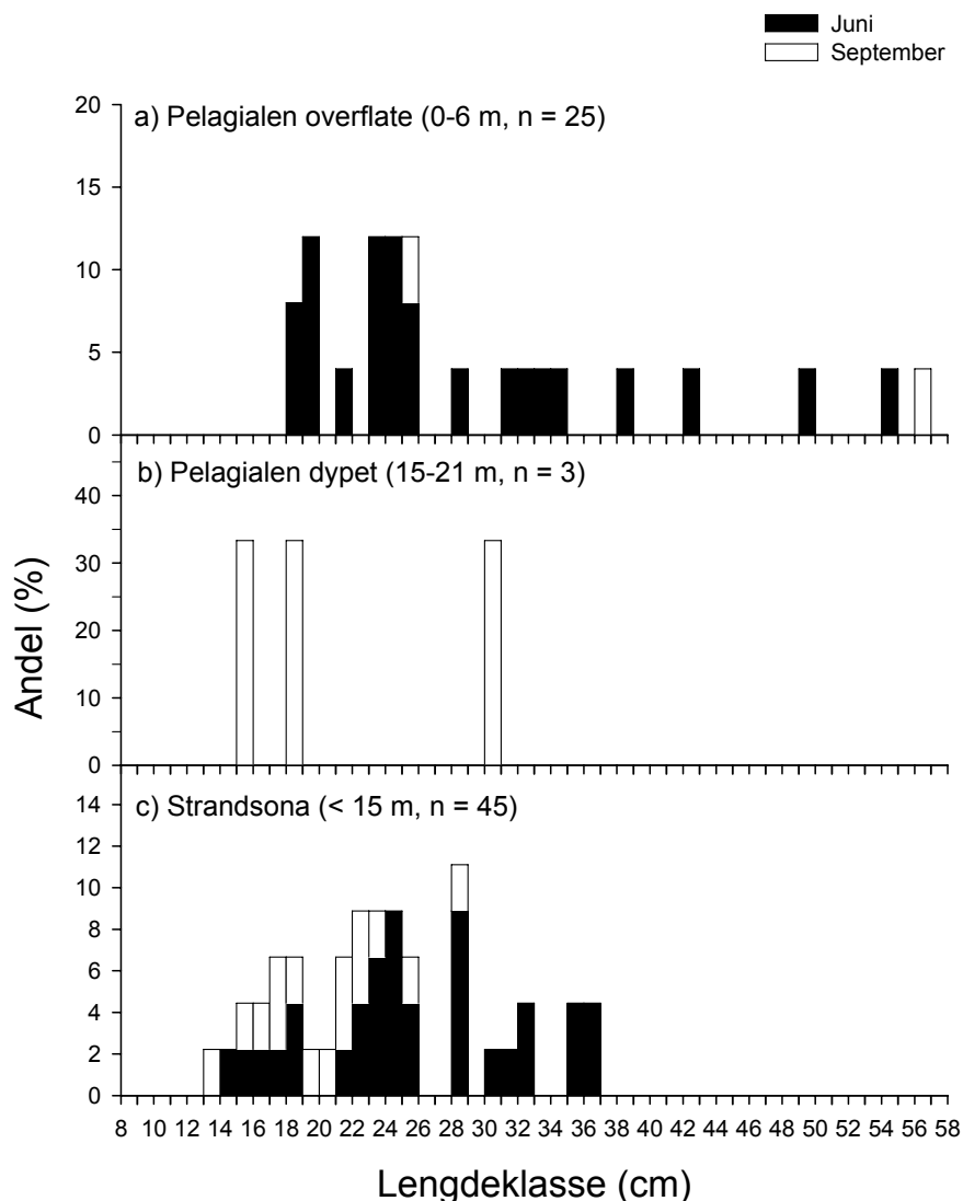
Figur 4.12 Lengdefordeling til ørret fanget på flytegarv på a) 0-6 m dyp og b) 15-21 m dyp og med bunngarv i c) strandsona. (Det ble ikke fanget ørret på bunngarv i profundalen, > 15 m).
