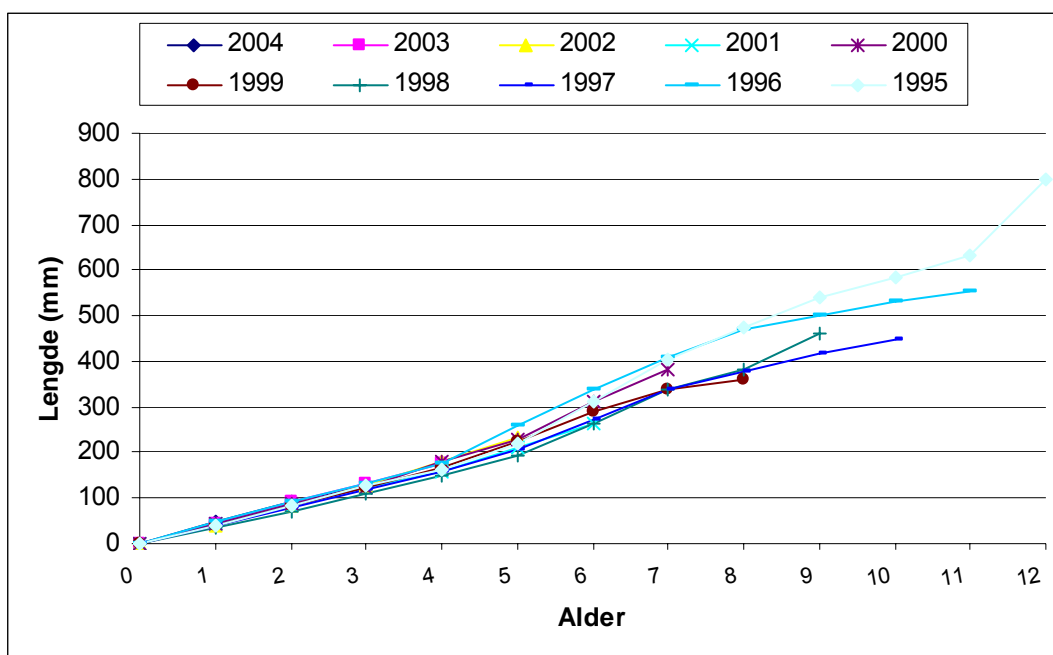
Figur 4.16 Tilbakeberegnet lengde for ulike årsklasser av umerket ørret ( n=92 ) fanget i Storsjøen i 2006 og 2007.
