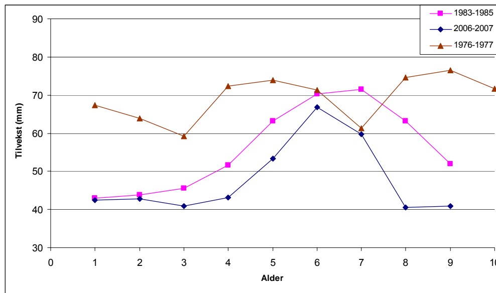
Figur 5.3 Beregnet gjennomsnittlig årlig tilvekst for ulike aldersklasser av ørret i Storsjøen i periodene 1976-77, 1983-185 og i 2007.
