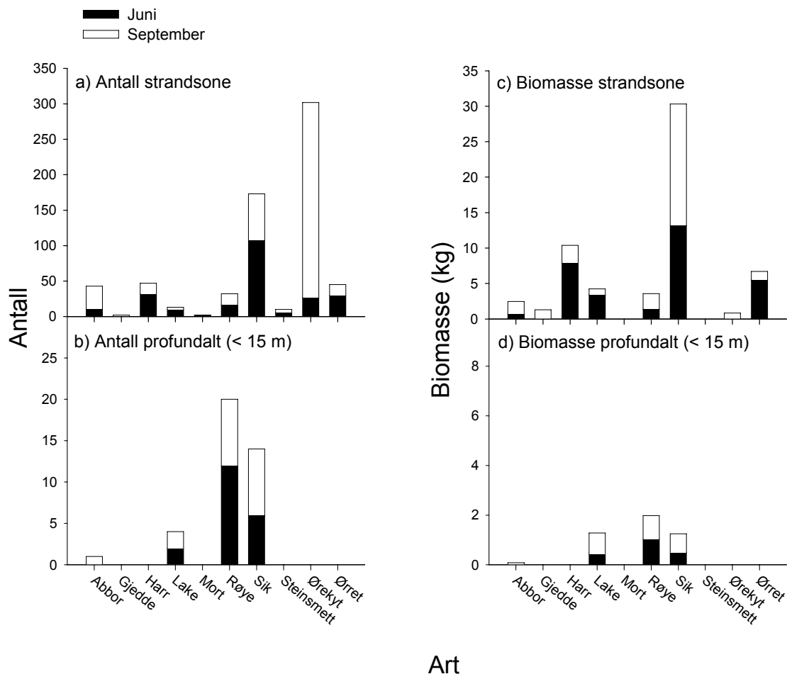
Figur 4.2 Bunnfiskfangster i antall og biomasse fordelt på strandsone og profundalsone (< 15 m). a) antall strandsone, b) antall profundalsone, c) biomasse strandsone og d) biomasse profundalsone. Prøvefiske i Storsjøen, juni og september 2007.
