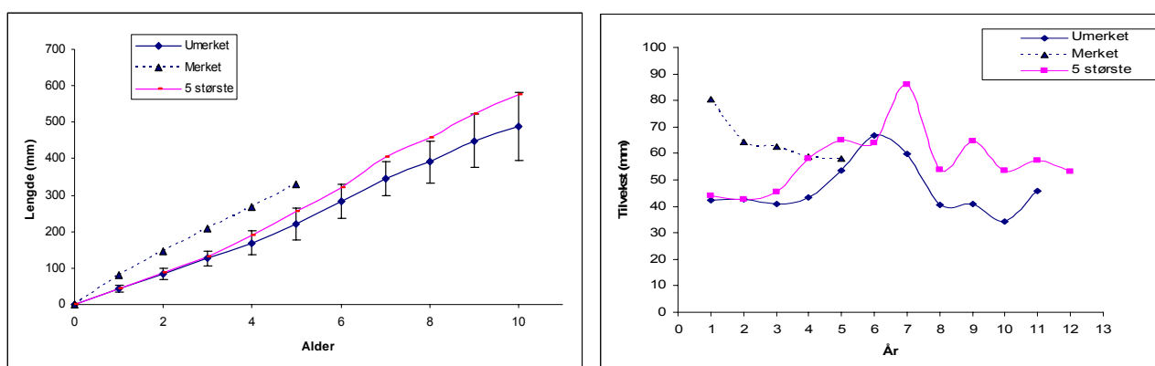
Figur 4.15 Tilbakeberegnet lengde (venstre, med \pm sd for umerket ørret) og årlig tilvekst (høyre) for umerket ørret ( n=92 ), merket ørret ( n=10 ) og de fem største ørretene som ble fanget/samlet inn i Storsjøen i 2006/2007.
