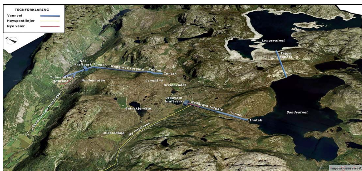
Figur 1. Skisse over tiltaket med røyrgater, tunnellar og kraftstasjonar (Lyse produksjon)
