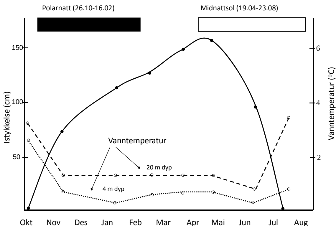
Figur 2 Sesongmessig variasjon i daglengde, istykkelse (heltrukken linje) og vanntemperatur (brukte linjer) i Linnévatn, Svalbard (1995-96).
