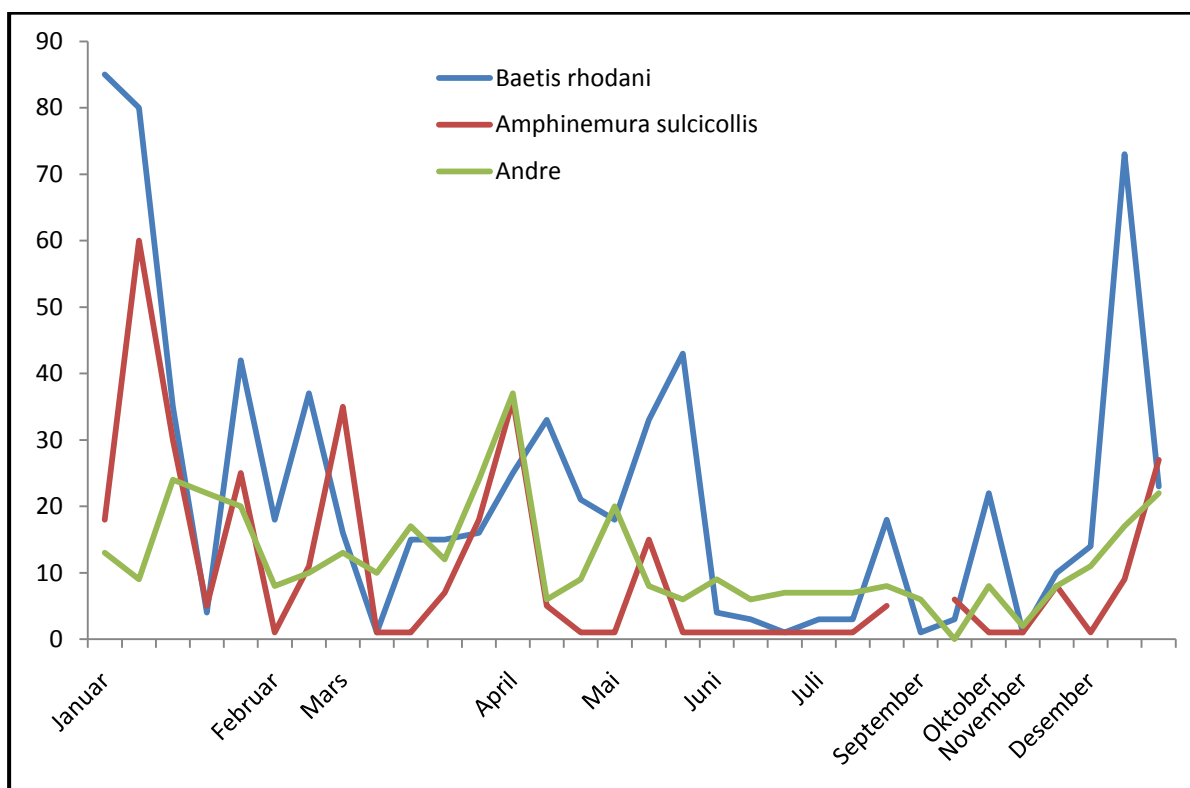
Figur 24. Sesongmessig variasjon i forekomst av de dominerende bunndyrtartene Baetis rhodani og Amphinemura sulcicollis samt 29 andre bunndyrtaksa i perioden 2006-2010. Verdiene er oppgitt som antall individer per minutt sparkeprøve.
