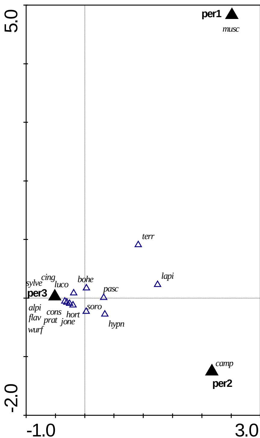
Figur 13. CCA-biplot av humler og periode (1, 2 og 3). Artene er beskrevet med de fire eller fem første bokstavene i artsnavnet (se Figur 3 for hele artsnavn).
