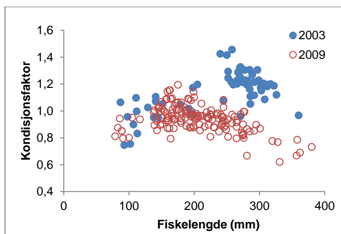
Figur 7. Kondisjonsfaktoren hos auren i Langevatn i 2003 og 2009.
