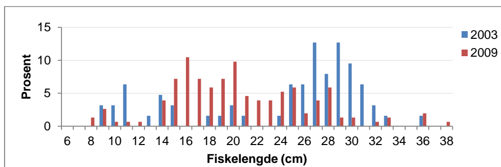
Figur 6. Lengdefordelingen hos auren i Langevatn i prøvfiskefangstene fra 2003 og 2009.
