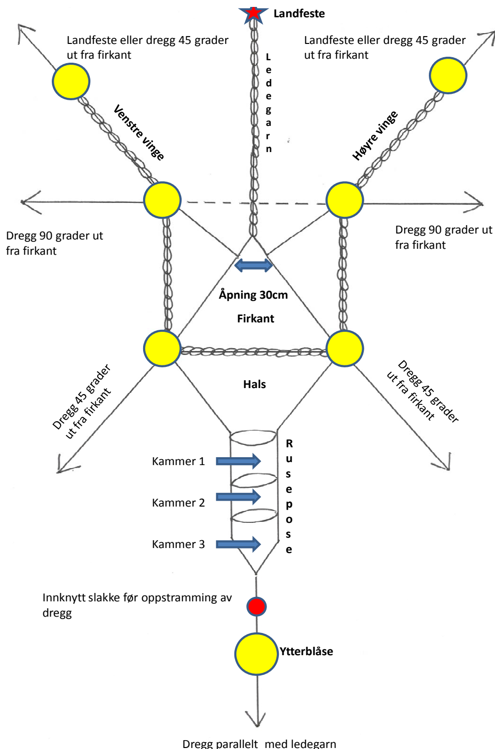
Figur 2. Skissetegning av "sjørretruse" sett ovenfra. Rusen består av fem hoveddeler; 1. Ledegarn (50m), 2. Firkant (5m*5m), 3. Vinger (2*10m), 4. Hals og 5. Rusepose med tre kammer. Fisk som møter ledegarnet/vingene vil følge dette inn i mot firkanten og videre gjennom halsen og inn i selve ruseposen. Hvert kammer har glidelåser som forenkler røkting og forhindrer tap av lus. Inngangen til ruseposen er sikret med en selsperre (skisse: Marius Berg).
