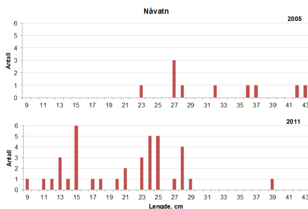
Figur 13. Lengdefordelingen hos auren i Nåvatn basert på prøvafiskefangstene fra 2005 og 2011.
