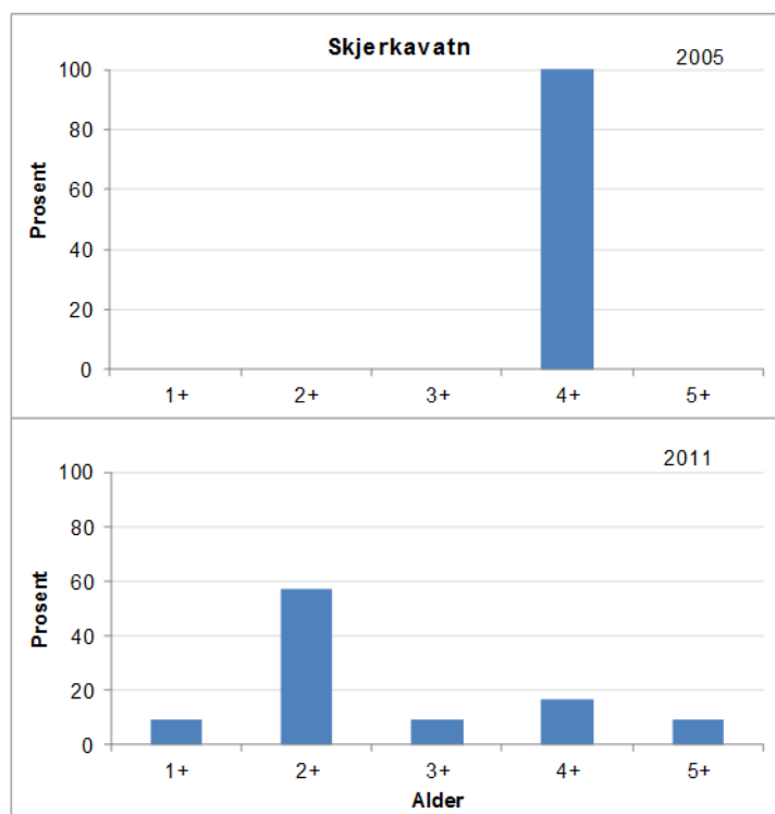
Figur 12. Aldersfordelingen hos aure i prøvafiskefangstene fra Skjerkevattn i 2011.
