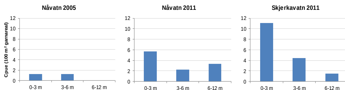
Figur 10. Garnfangster av aure i ulike dyp i Nåvatn (2005 og 2011) og Skjerkevatn (2011).
