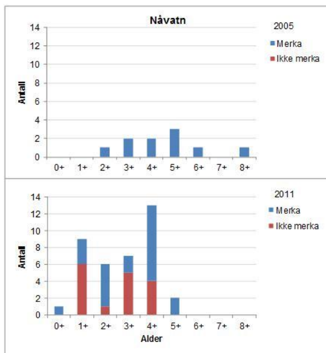
Figur 11. Aldersfordeling hos vill og utsatt aure i prøvofiskefangstene med garn fra Nåvatn i 2005 og 2011.
