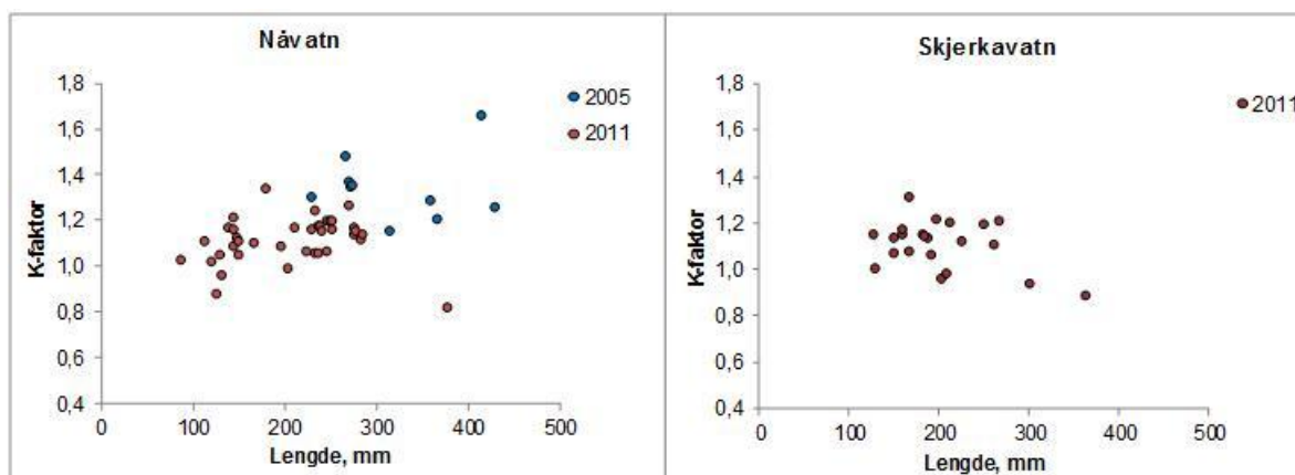
Figur 15. Kondisjonsfaktoren hos auren i Náváttn i 2005 og 2011 og i Skjerkevatn i 2011 sett i forhold til fiskens kroppslengde.
