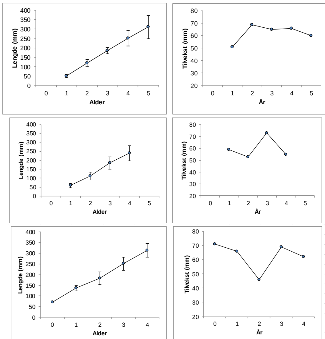
Figur 14. Tilbakeberegnet lengde (venstre) og tilvekst (høyre) hos auren i Nåvatn i 2005 (øverst), Nåvatn 2011 (midten) og Skjerkevattn 2011 (nedst).
