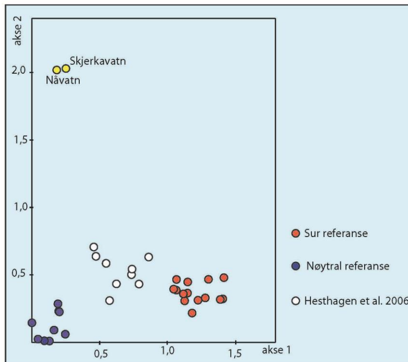
Figur 8. Aktiv DCA-ordinasjon av krepsdyrfaunaen (forekomst/fravær) i Nåvatn og Skjerkavatn samt i ni andre sørlandslokaliteter (Hesthagen mfl. 2006) og åtte nøytrale innsjøer som benyttes som referanselokaliteter.
