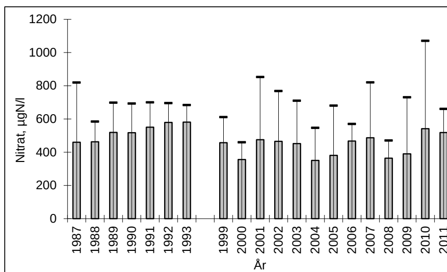
Figur 6. Årsgjennomsnitt (søylor) og maksimumsverdier for nitrat ( \text{NO}_3 , µg/l) ved Lindtjørnhølen for 1987-1993 og 1999-2011.
