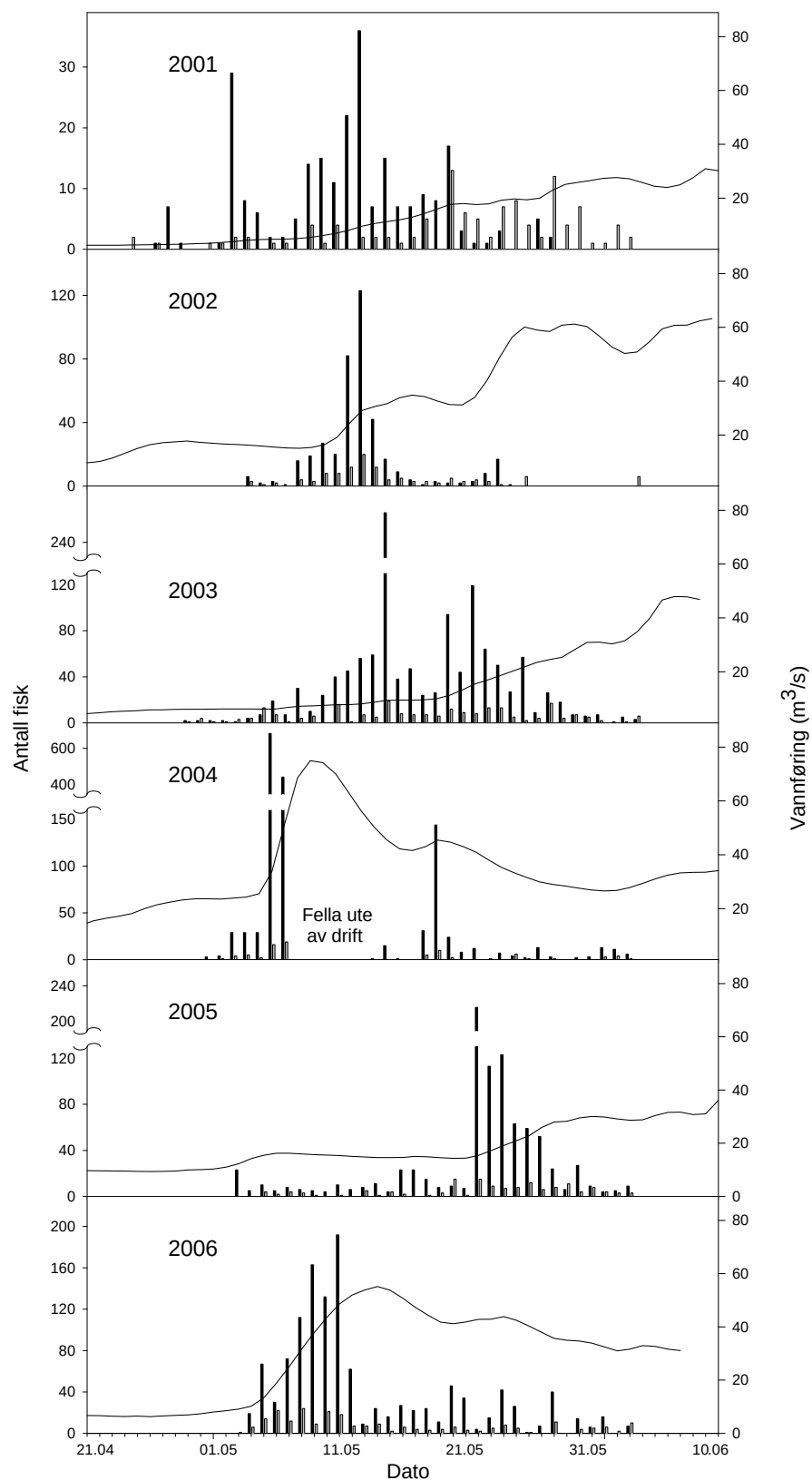
Figur 9a. Fangster av villsmolt av laks (svarte stolper) og sjøørret (hvite stolper) i smoltfella i Eira, samt vannføring (kurve) i årene 2001-2006.
