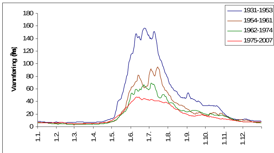
Figur 4. Gjennomsnittsvannføring i Eira før utbygging (1931-1953), etter Aurlautbyggingen (1954-1961), etter Takrenna (1962-1974) og etter Gryttenreguleringen (1975-2007).
