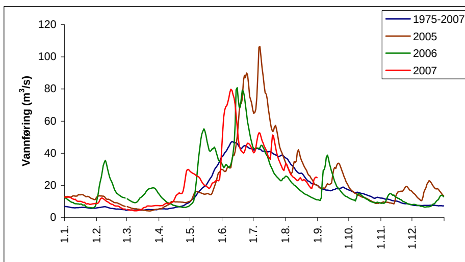
Figur 5. Gjennomsnittsvannføring (døgnsnitt) i Eira (m 3 /s) for perioden etter Gryttenreguleringen (1975-2007), samt døgnsnittsvannføring for 2005, 2006 og 2007. Data fra NVE.
