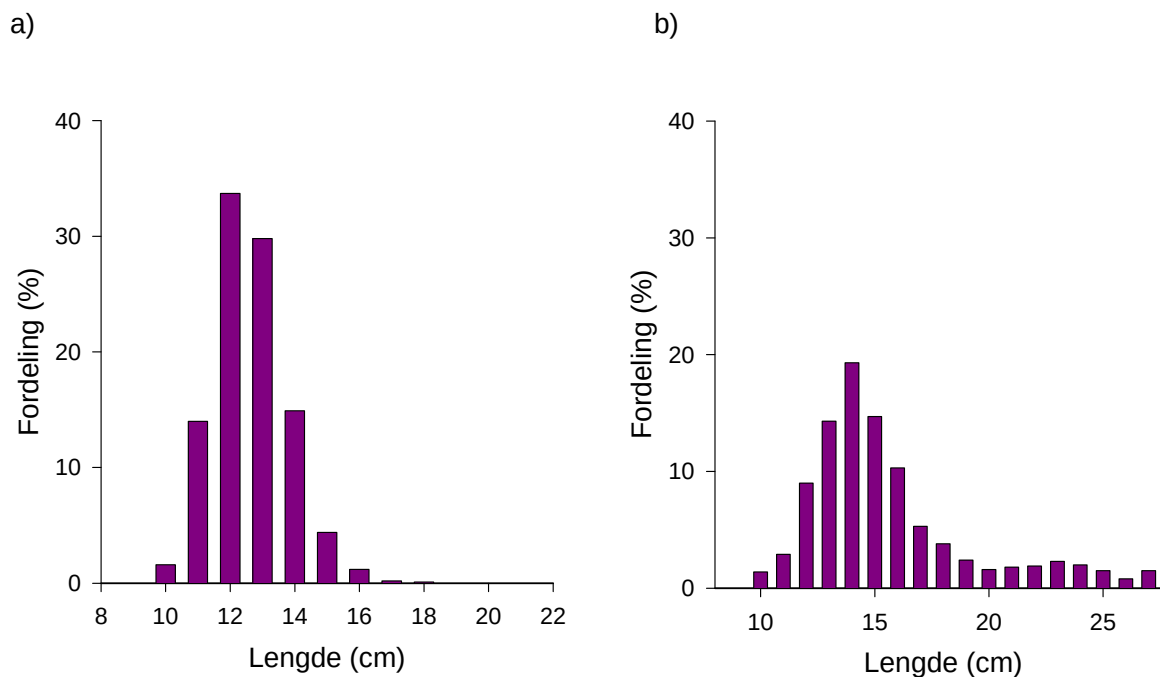
Figur 10. Lengdefordeling av villsmolt av a) laks og b) sjørøtt som vandret ned i smoltfella i Eira i årene 2001-2007. Antall: 6 332 laks og 989 ørret.
