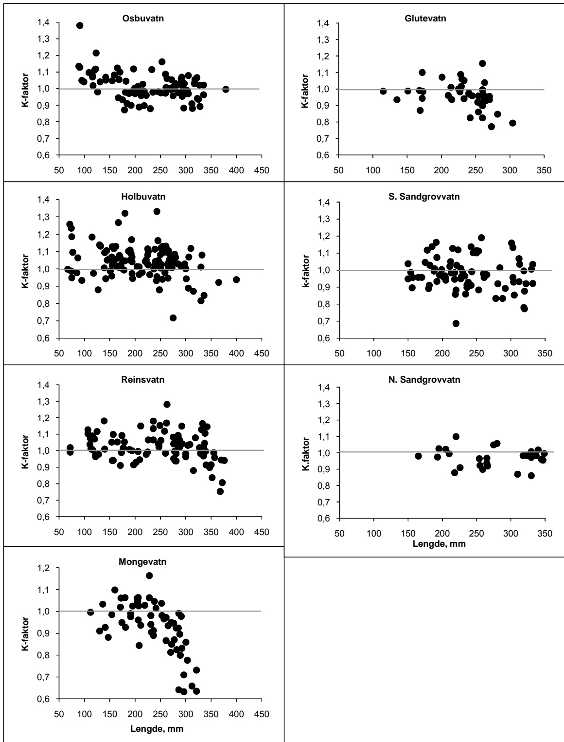
Figur 14. Kondisjonsfaktor i forhold til lengden hos auren i de enkelte innsjøene. De horisontale linjene angir verdien 1,0.
