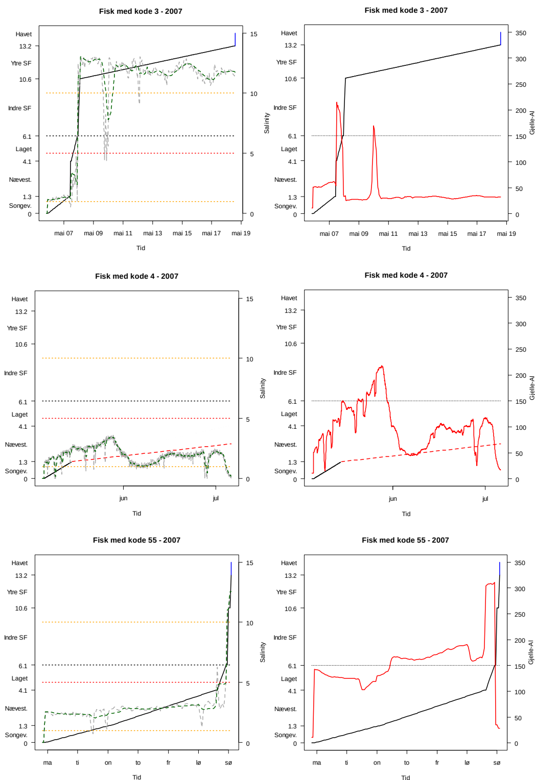
Figur 17. Noen utvalgte smolt fra 2007 med forskjellig utvikling. Venstre panel gir utvandring mot simulert salinitet, mens høyre panel gir utvandring mot predikert Gjelle-Al nivå. Venstre vertikal akse viser distansen utover i fjordsystemet. Den hele, svarte linja i venstre panel angir smoltens utvandringshistorie, mens de grå og grønne stiplede linjene angir simulert salinitet for sone og tidsperiode (grå gir samtidig timevis salinitet mens den grønne gir saliniteten midlet over de siste 12 timene). Rød horisontal stiplede linje angir Salinitet lik 5 ppt ("verste" nivå), mens de oransje stiplede linjene gir Salinitet hhv. lik 1 og 10 ppt. I høyre panel er telemetriregistreringene plottet på samme måte som tidligere mens den røde heltrukne linja angir predikert Gjelle-Al for 12 timers midlet salinitet.
