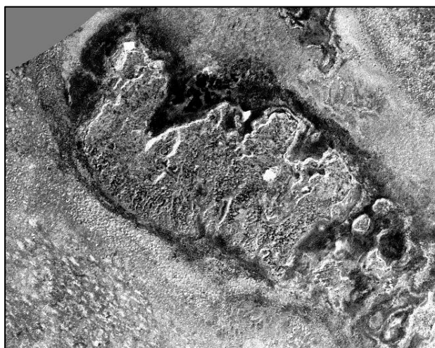
Figur 14. Endringsbilde ved hjelp av PCA-analyse av de pankromatiske bildene fra 2004 og 2010. De lyse og hvite områdene indikerer at forandringer har skjedd i bildet, som forandringer i pøler, bruddkanter, sprekker og naken torv.
